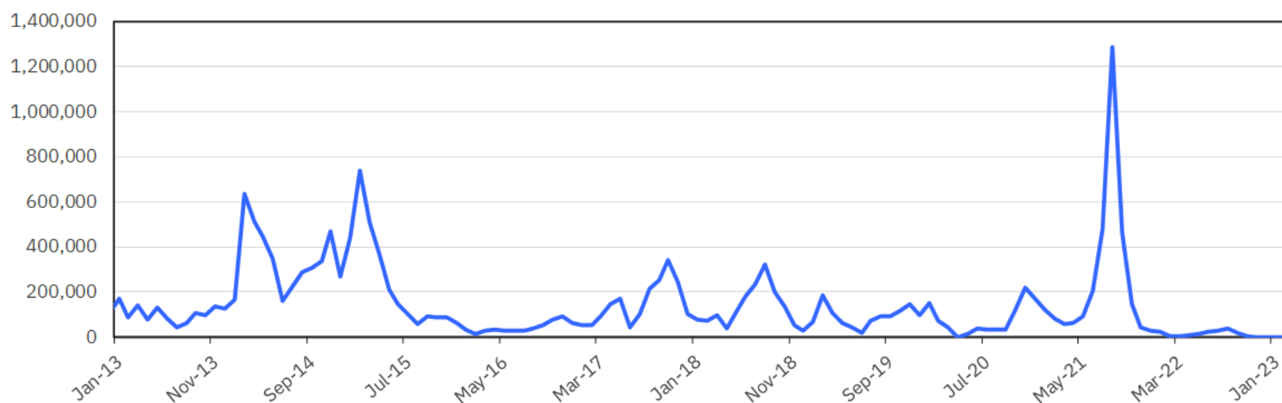
Custo Marginal de Operação Agregado - Brasil (Agregado CMO x Carga Verificada)
