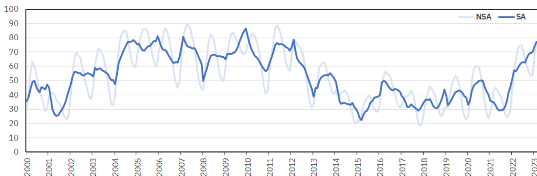
EAR - Energia Armazenada - Brasil (% do potencial)
