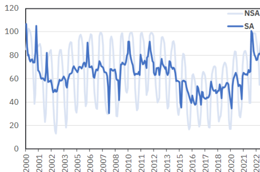
EAR - Sistema Norte (% do potencial)
