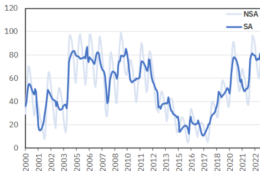
EAR - Sistema Nordeste (% do potencial)
